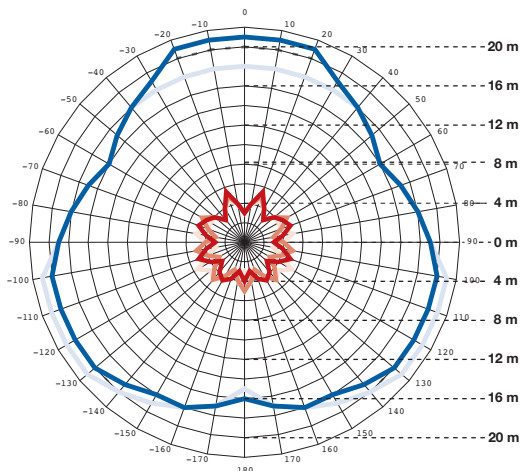
Rekkevidde IS 3360, Finjustering ved å forskyve linsen (blå = tangential gåretning, rød = radial gåretning)
